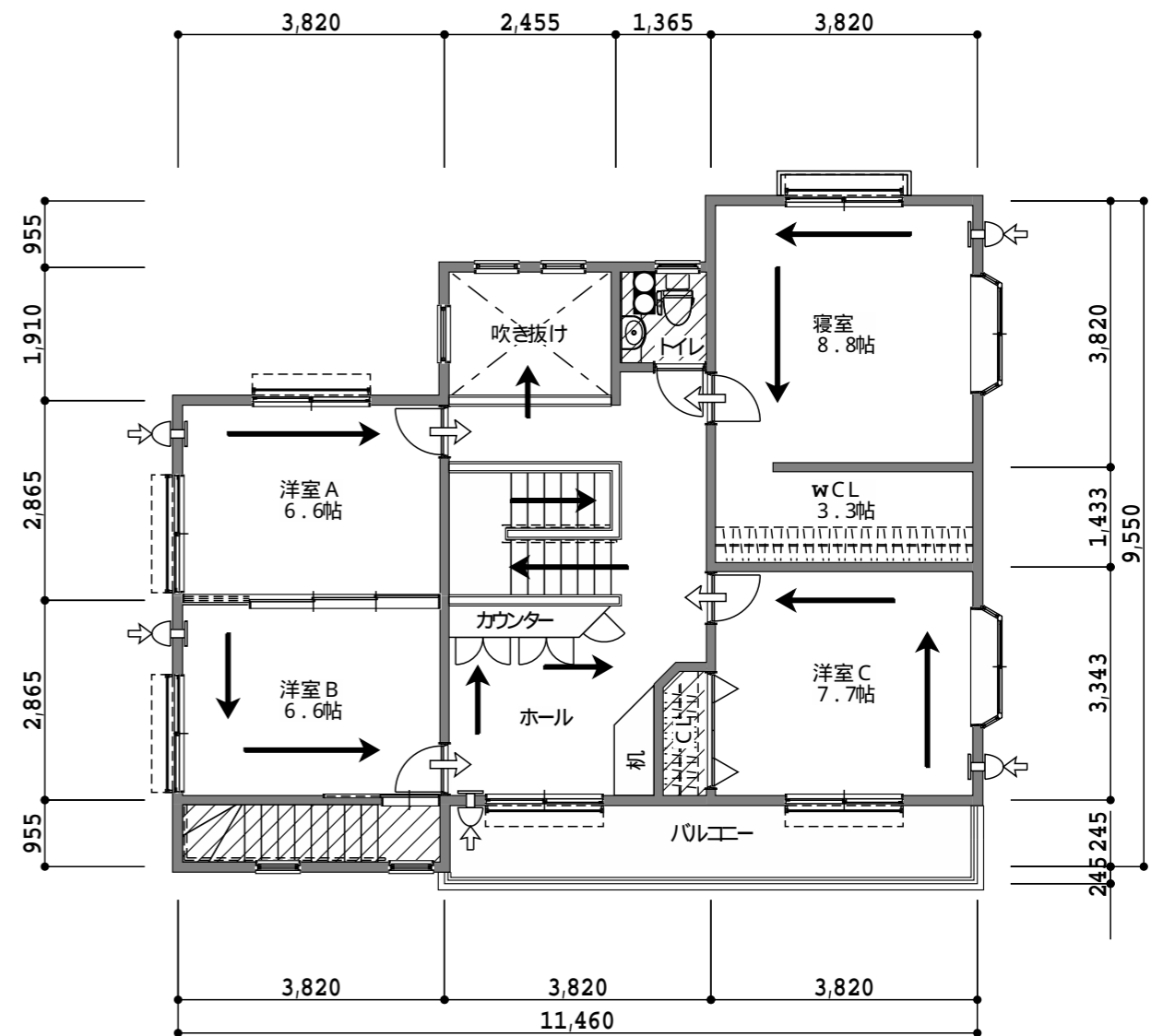
2階平面図
