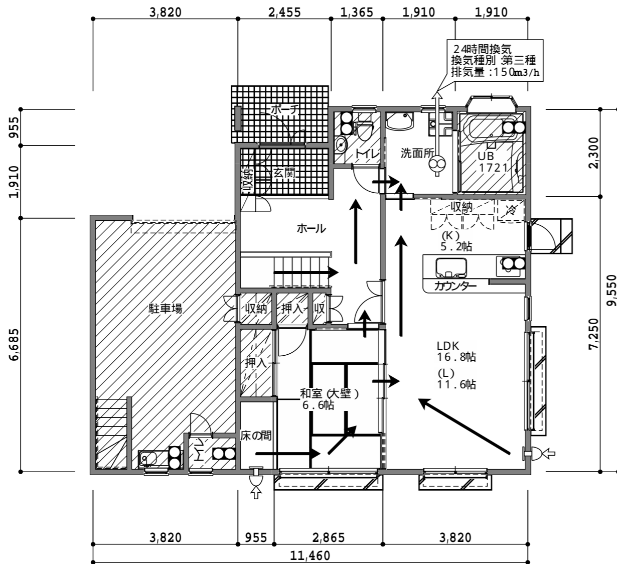
1階平面図
