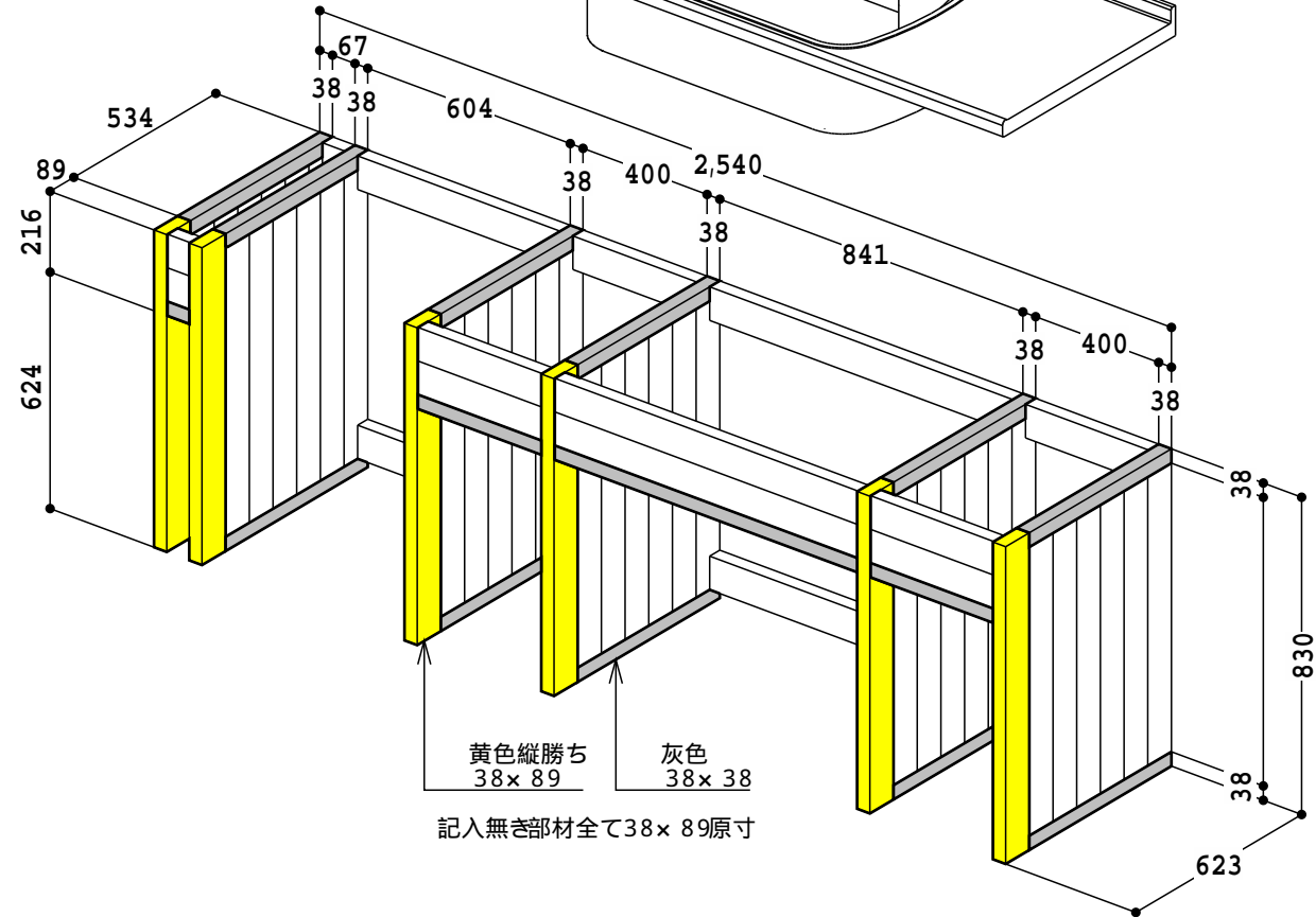
キッチン制作図
