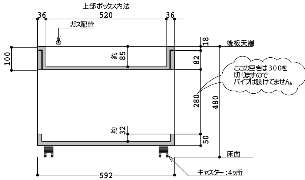
ワゴン断面図
