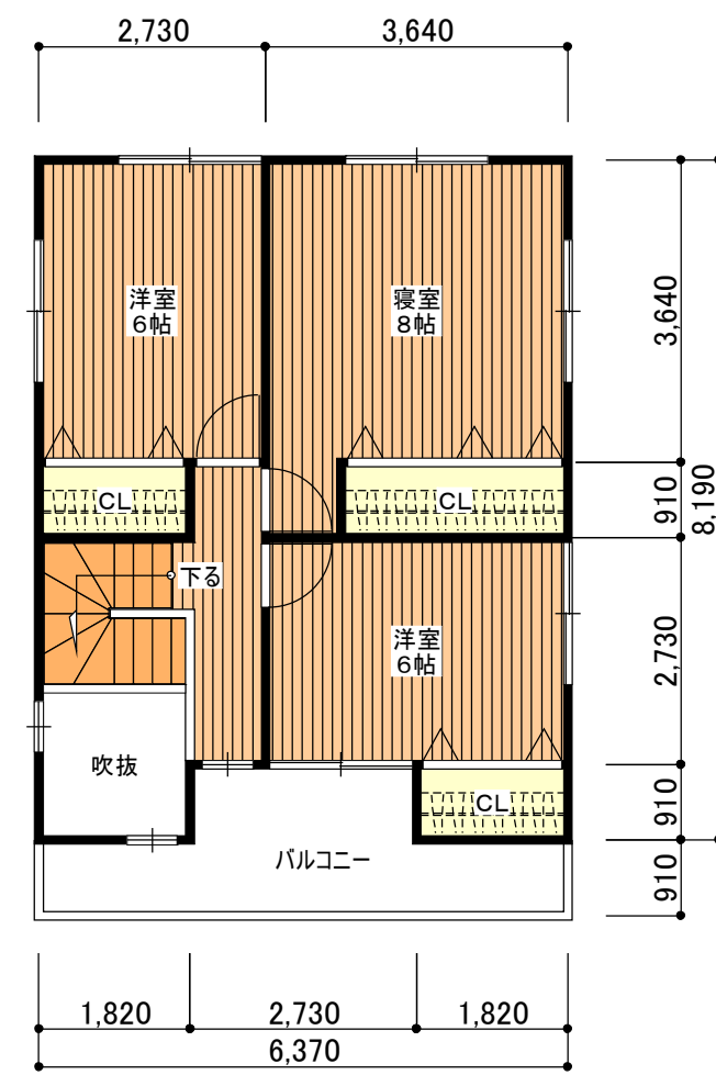
2階平面図-タイプB
