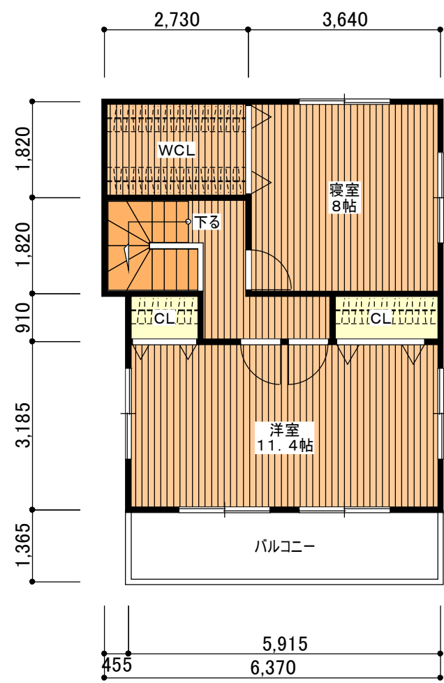
2階平面図-タイプA
