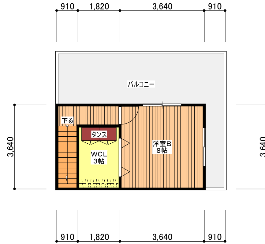
2階平面図
